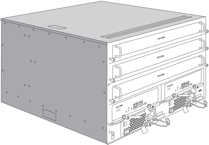
图1-6 TL-S7903设备外观（正面）
