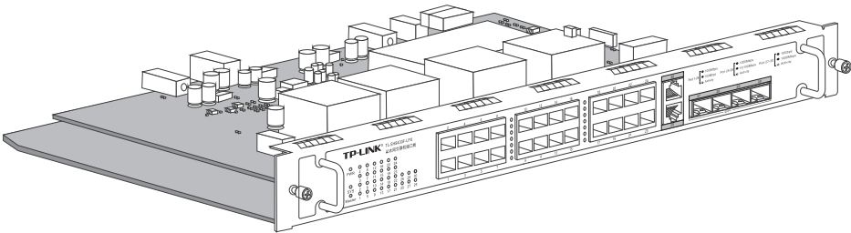
图1-18 TL-SH8430F-LPU业务板外观
