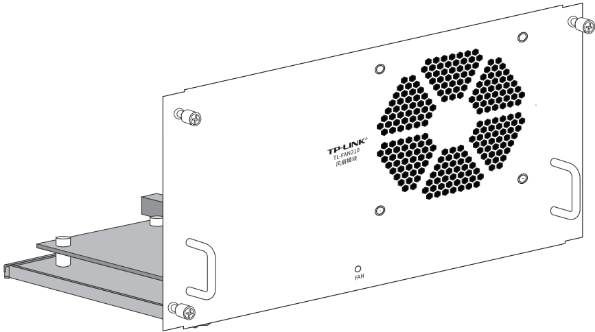
图1-28 TL-FAN210风扇模块外观
