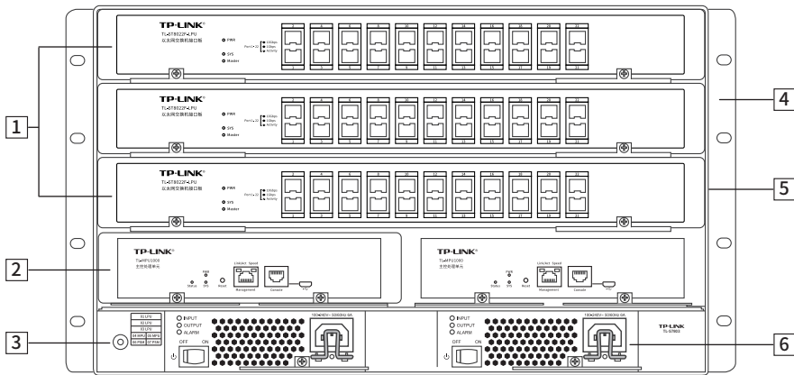
图1-8 TL-S7903机框结构示意图（正面）
