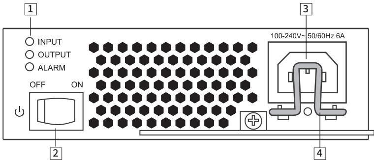
图1-25 TL-PSM800-AC结构示意图
