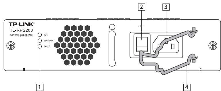
图1-23 TL-RPS200结构示意图
