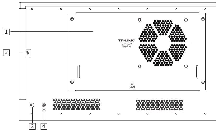
图1-9 TL-S7903机框结构示意图（背面）
