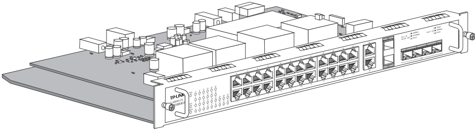
图1-14 TL-SH8430-LPU业务板外观
