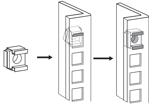
图2-3 浮动螺母安装示意图
