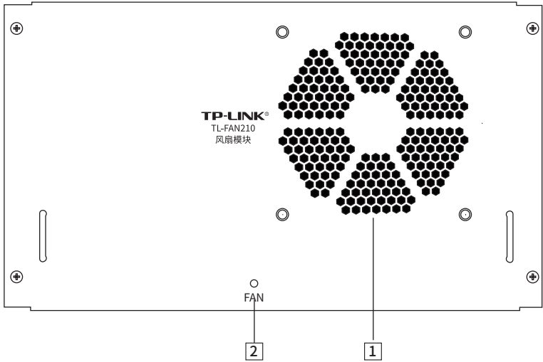
图1-29 TL-FAN210结构示意图
