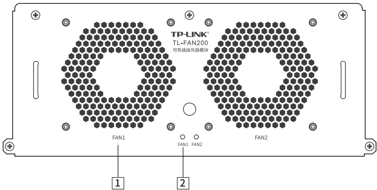
图1-27 TL-FAN200结构示意图
