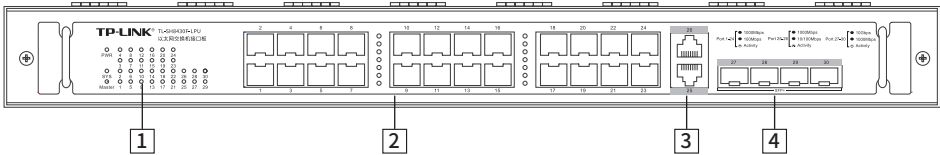
图1-19 TL-SH8430F-LPU结构示意图
